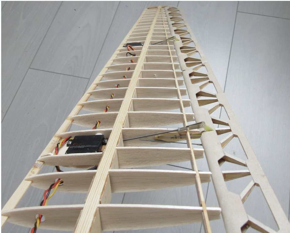
Two servos per aileron.
